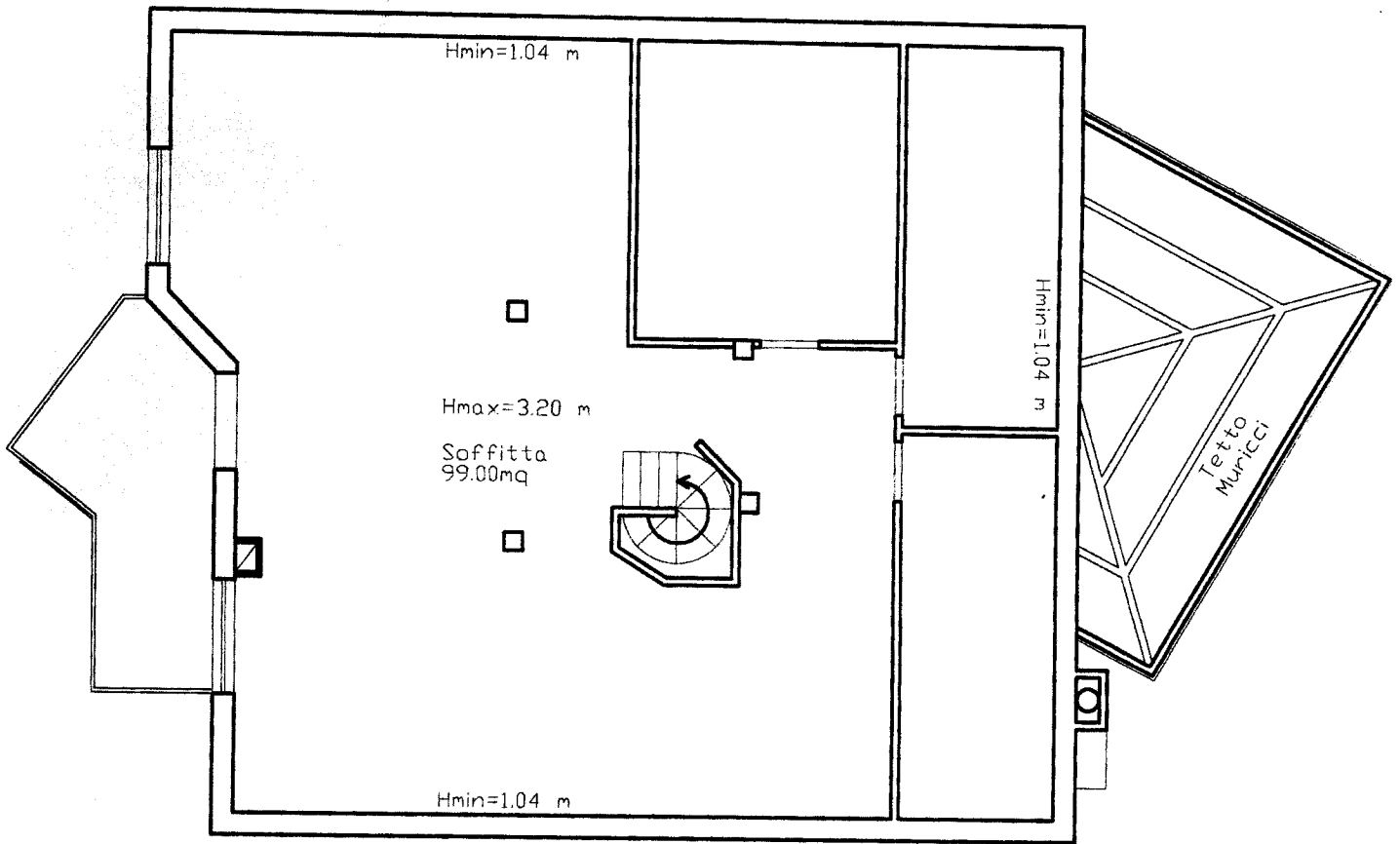
PIANO SOTTOTETTO
