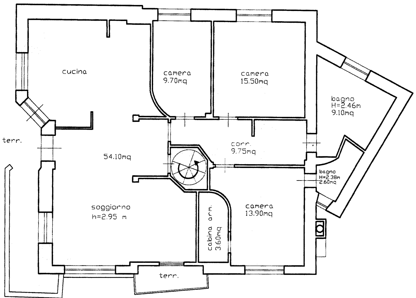
PIANO PRIMO
